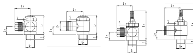
Limiteur de débit POM et Laiton nickelé
