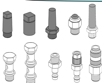
Raccords à coiffe
