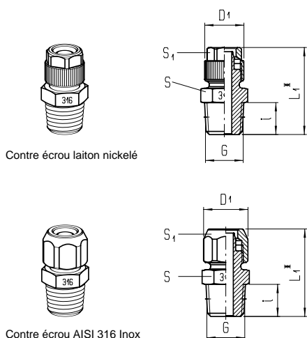
Contre écrou AISI 316 inox
